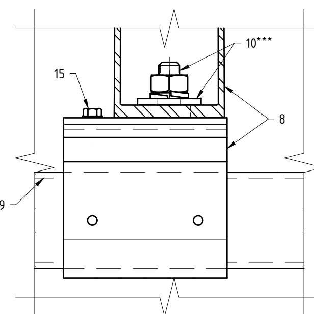
Модульная система: вид спереди (доп. вариант исполнения нижней петли)
