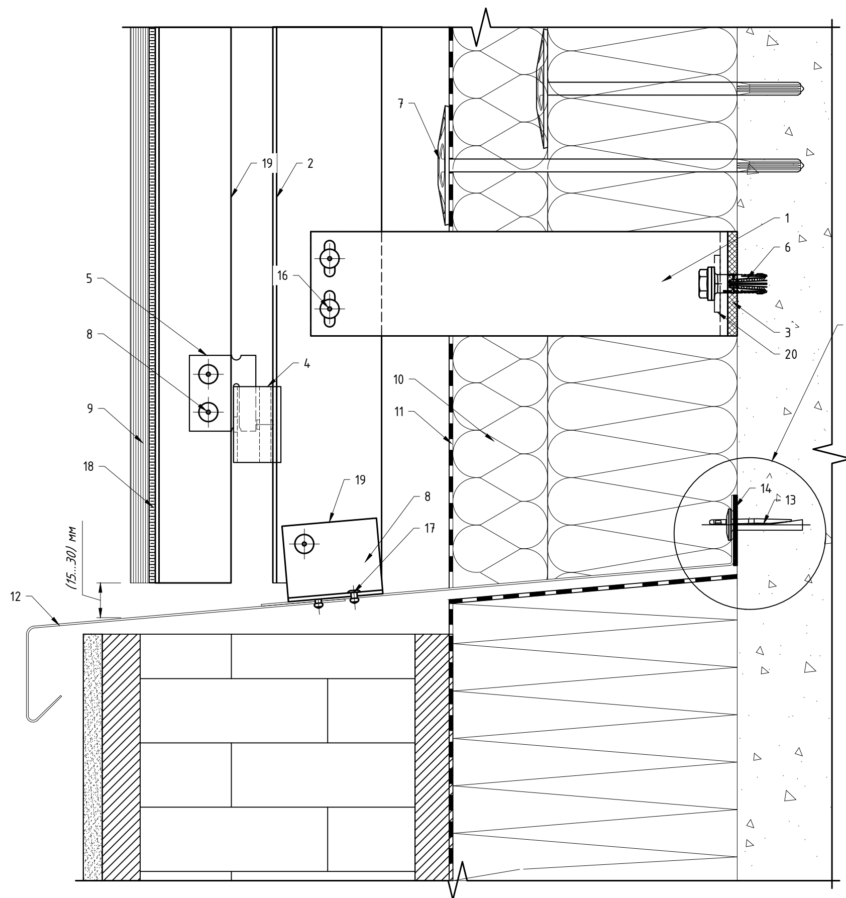
Вариант крепления отлива №1
