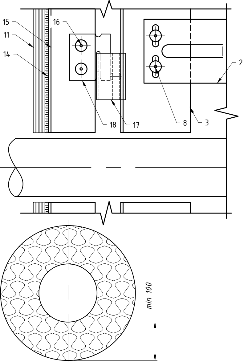
Крепление Rockpanel: вариант №2 (скрытое крепление, клей, клеящая лента, салазки и икли)
