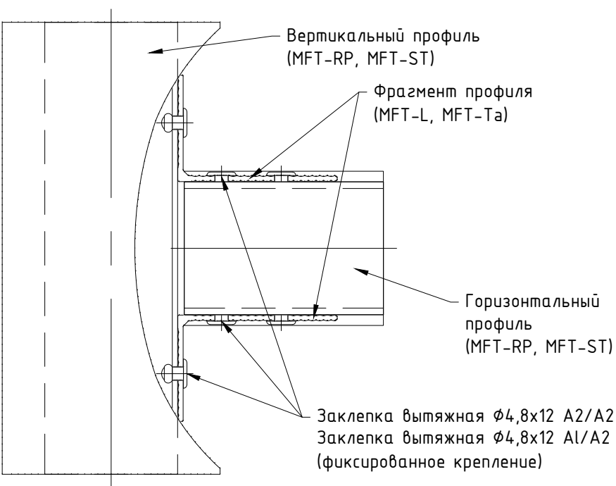
Узел №1 (увеличено)
