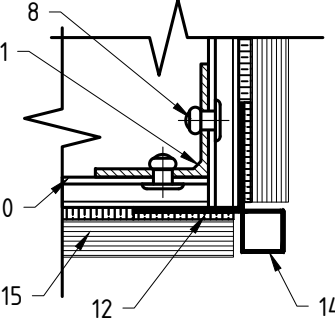
Крепление Rockpanel: вариант №4 (скрытое крепление, клей и клеящая лента)
