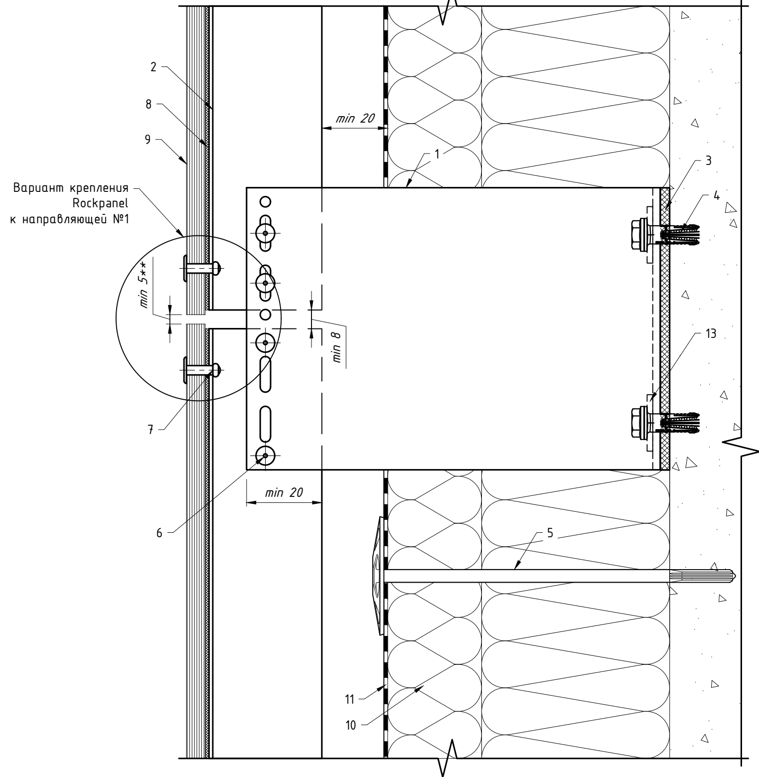
Вертикальный разрез: вариант №4.
