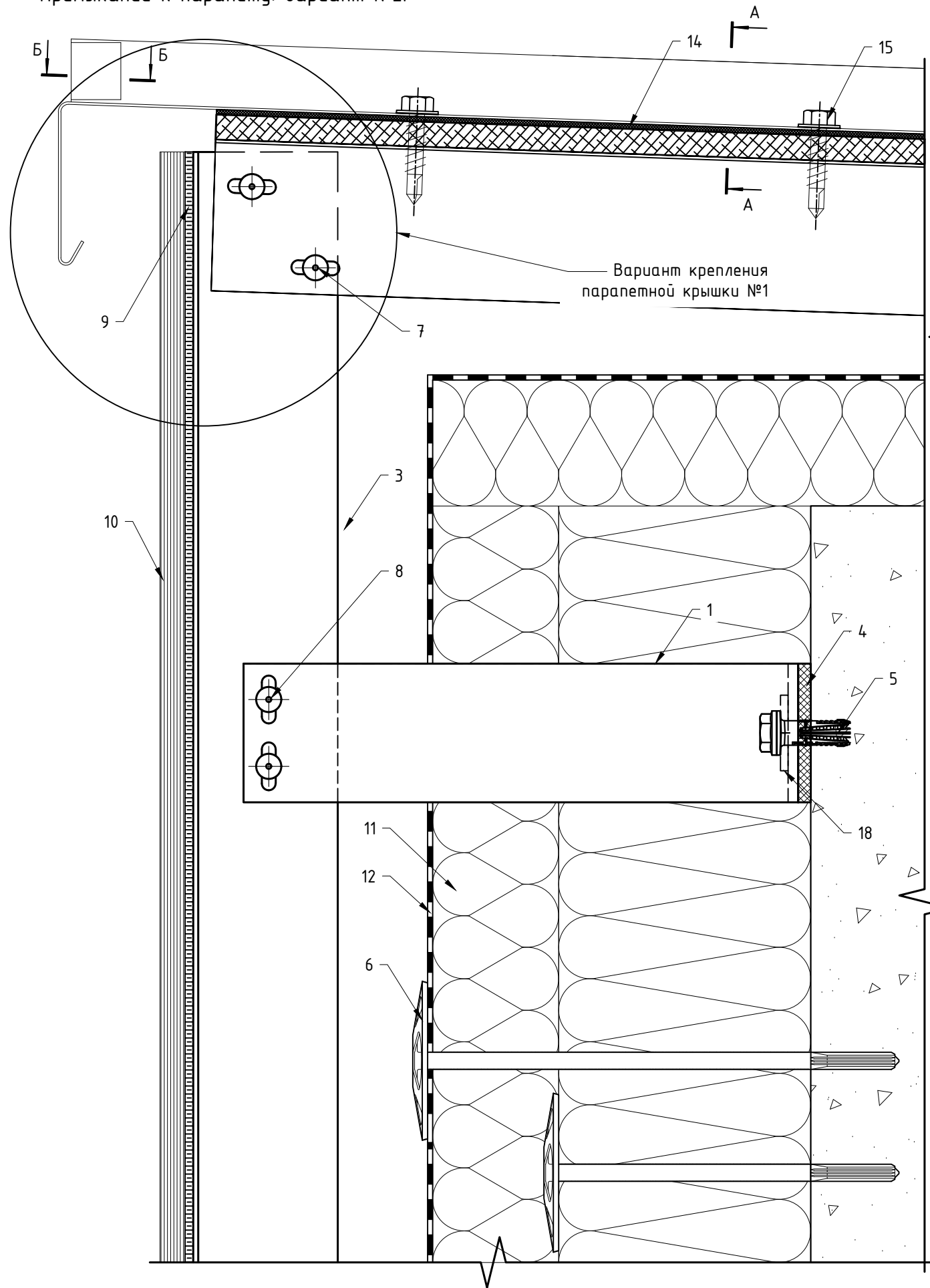
Примыкание к парапету: вариант №2.
