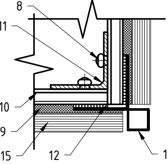
Крепление Rockpanel: вариант №2 (видимое крепление, заклепки)
