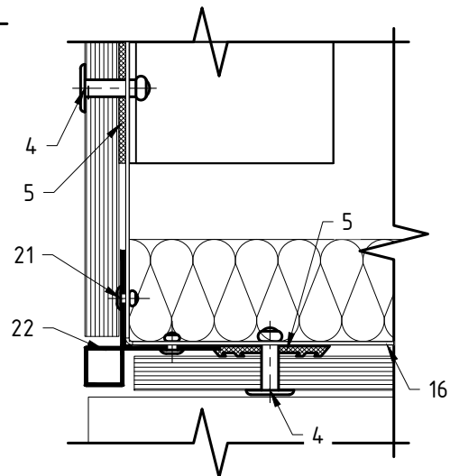
Вариант исполнения угла №2
