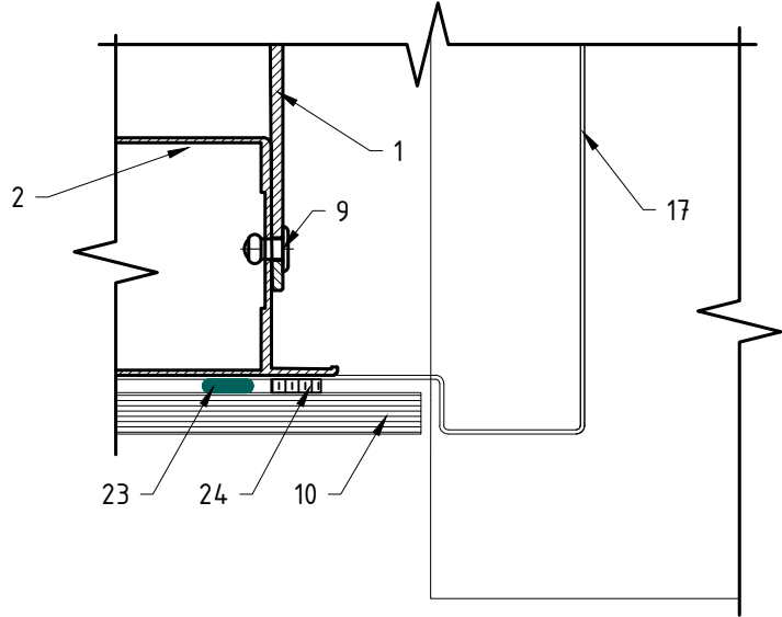
Вариант крепления Rockpanel к направляющей №2
