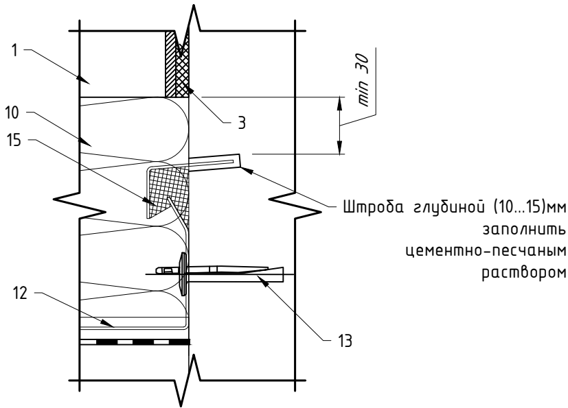
Вариант крепления оцинкованного листа №2
