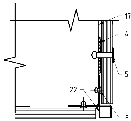
Вариант исполнения угла №2
