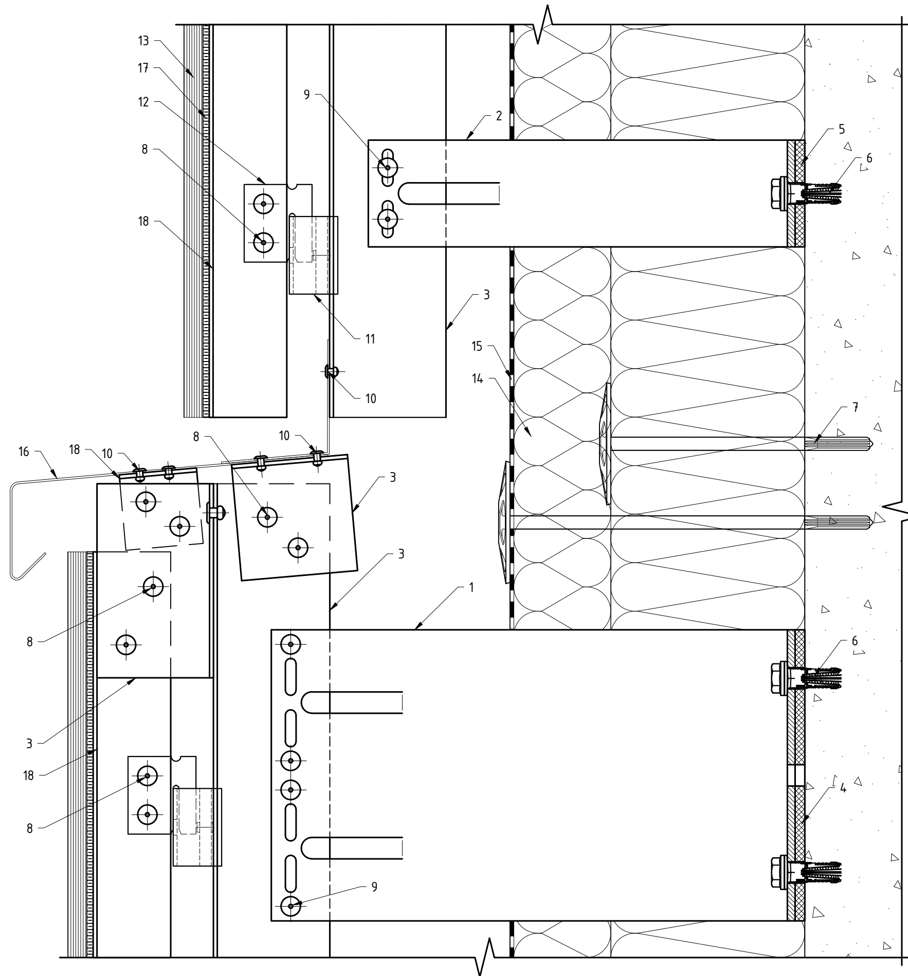
7.12 Организация перепада плоскостей облицовки: вариант №1. Крепление Rockpanel к направляющей: вариант 3.
