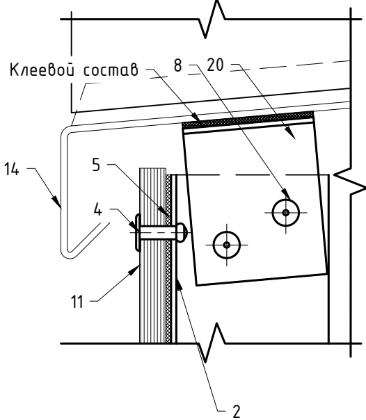
Вариант крепления отлива к направляющей №3
