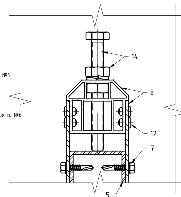
Модульная система: вид спереди (показано с регулировочным комплектом M12)
