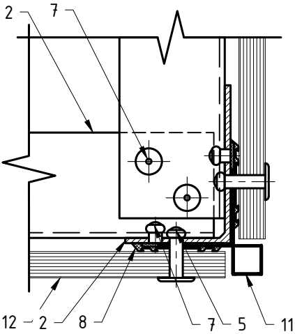
Крепление Rockpanel: вариант №2 (видимое крепление, заклепки)
