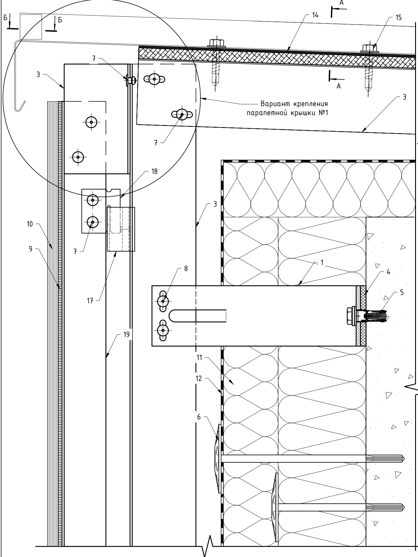
7.9 Примыкание к парапету: вариант №3.
