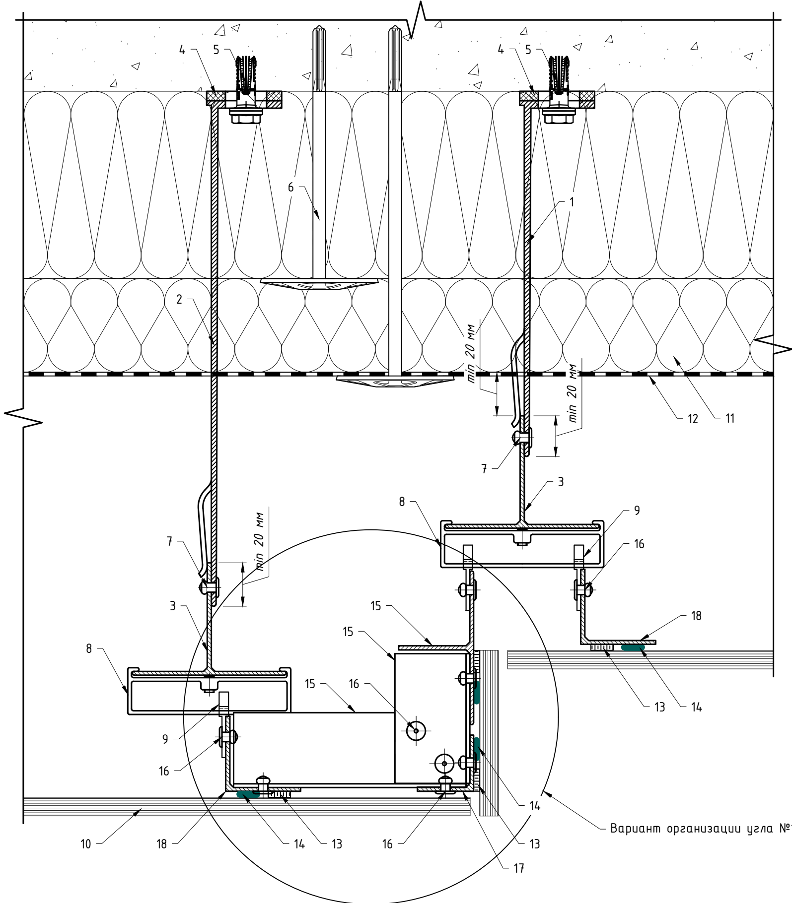
7.12 Организация перепада плоскостей облицовки: вариант №3. Крепление Rockpanel к направляющей: вариант 3.
