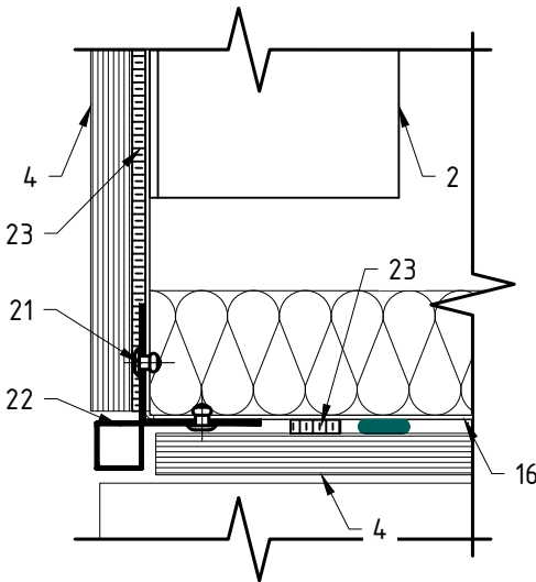
Вариант крепления Rockpanel к направляющей №2
