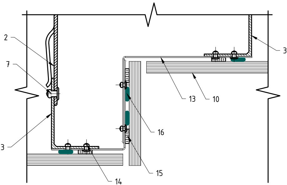
Крепление Rockpanel к направляющей: вариант №2
