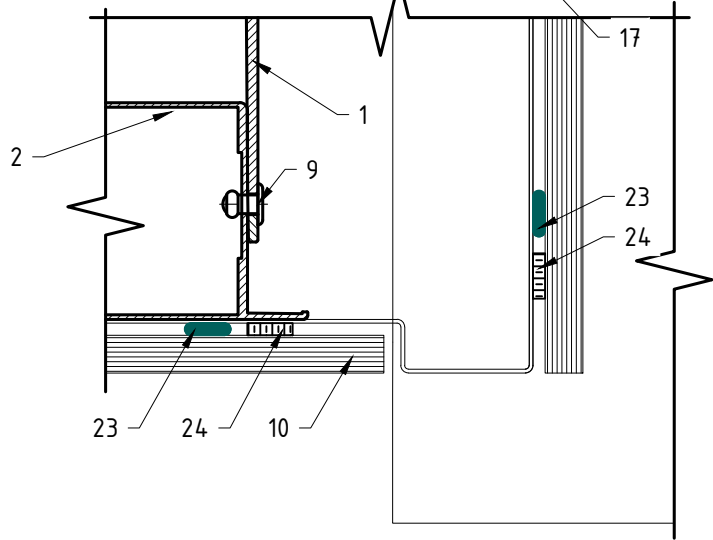
Вариант крепления Rockpanel к направляющей №2
