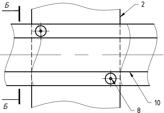
Крепление Rockpanel: вариант №2 (видимое крепление, заклепки)
