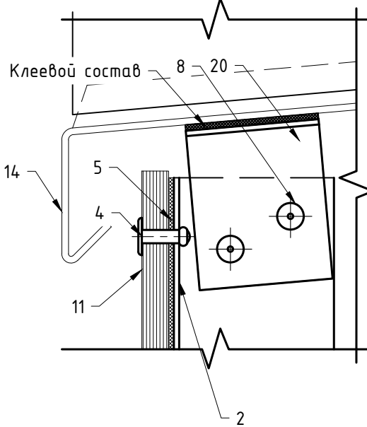
Вариант крепления отлива к направляющей №3
