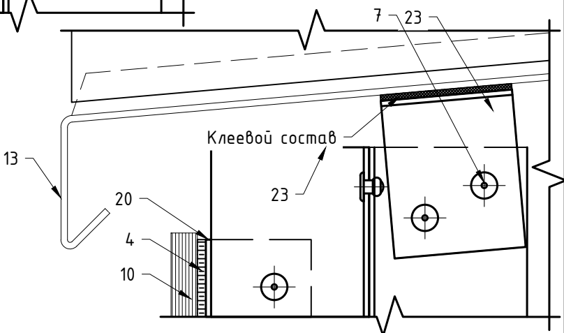
Вариант крепления отлива к направляющей №3
