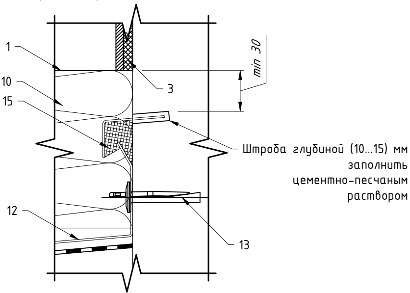
Вариант крепления отлива №2
