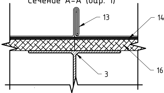
Сечение А-А (вар. 2)
