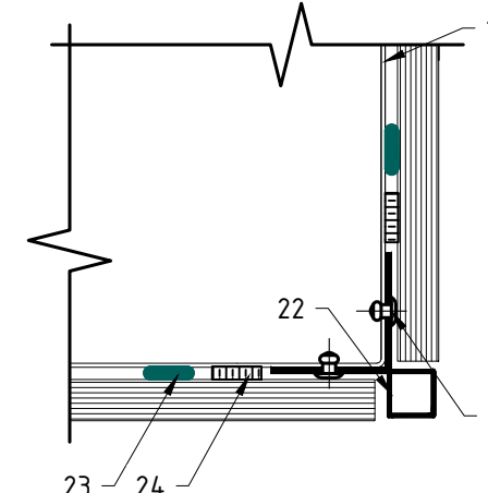
Вариант крепления Rockrapel к направляющей №2
