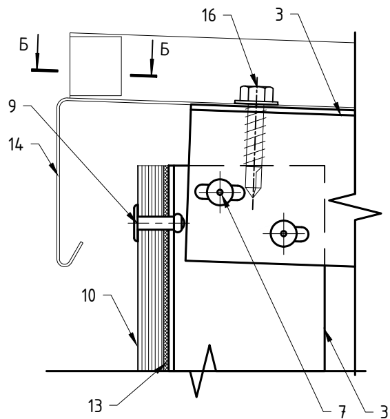
Сечение Б-Б (для варианта 1)
