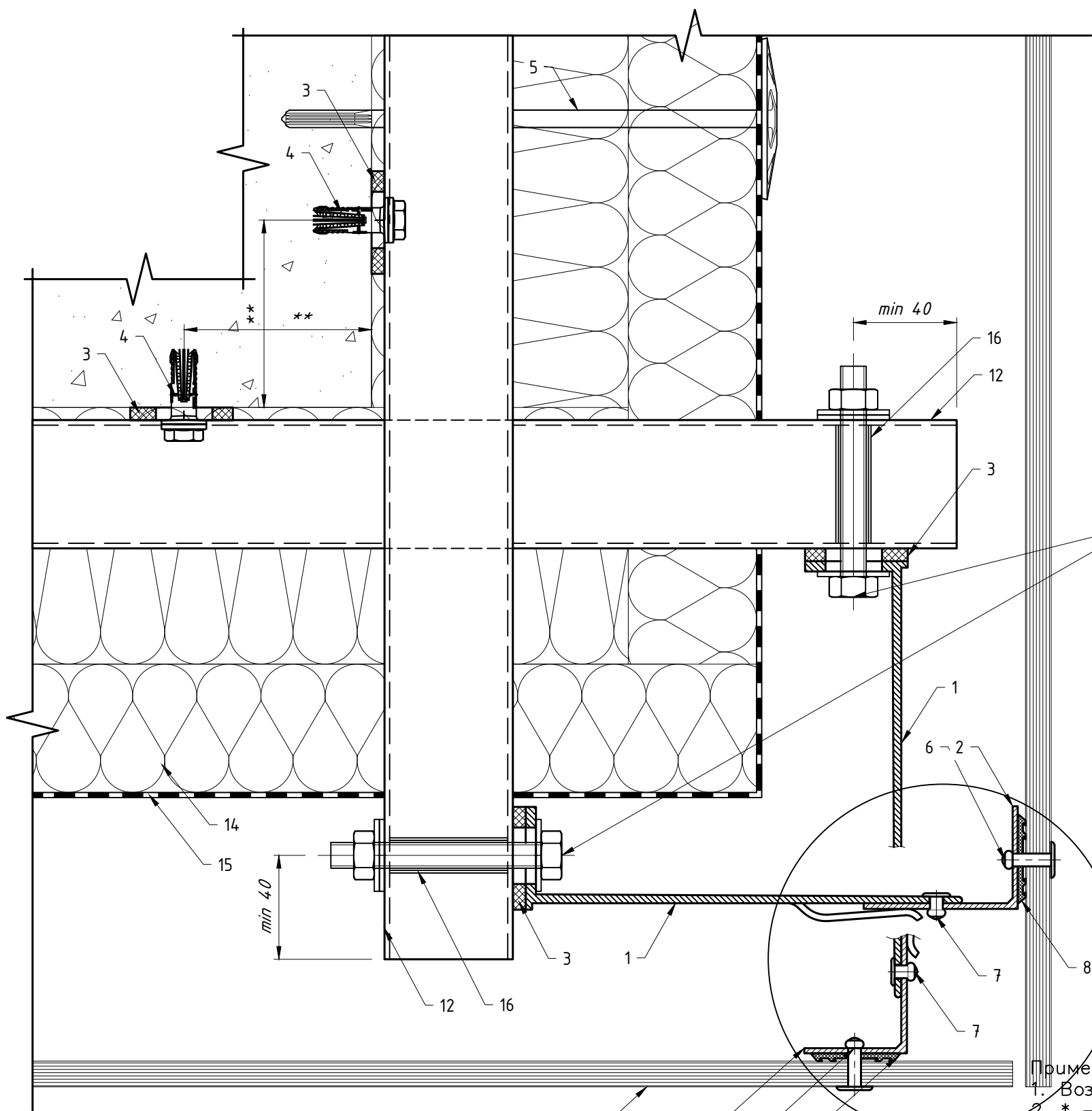
Крепление Rockpanel: вариант №1***
