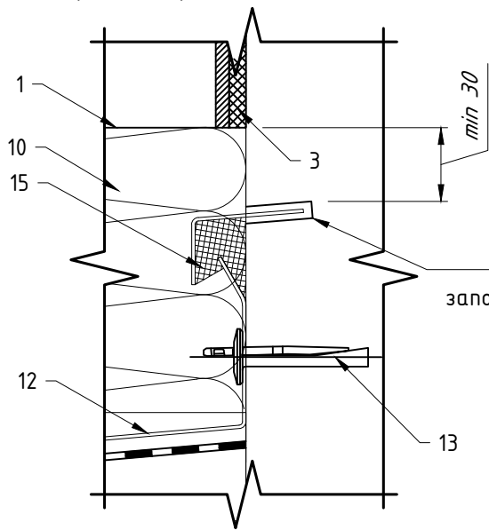
Вариант крепления отлива №2
