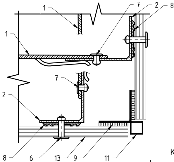
Крепление Rockpanel: вариант №2 (видимое крепление, заклепки)
