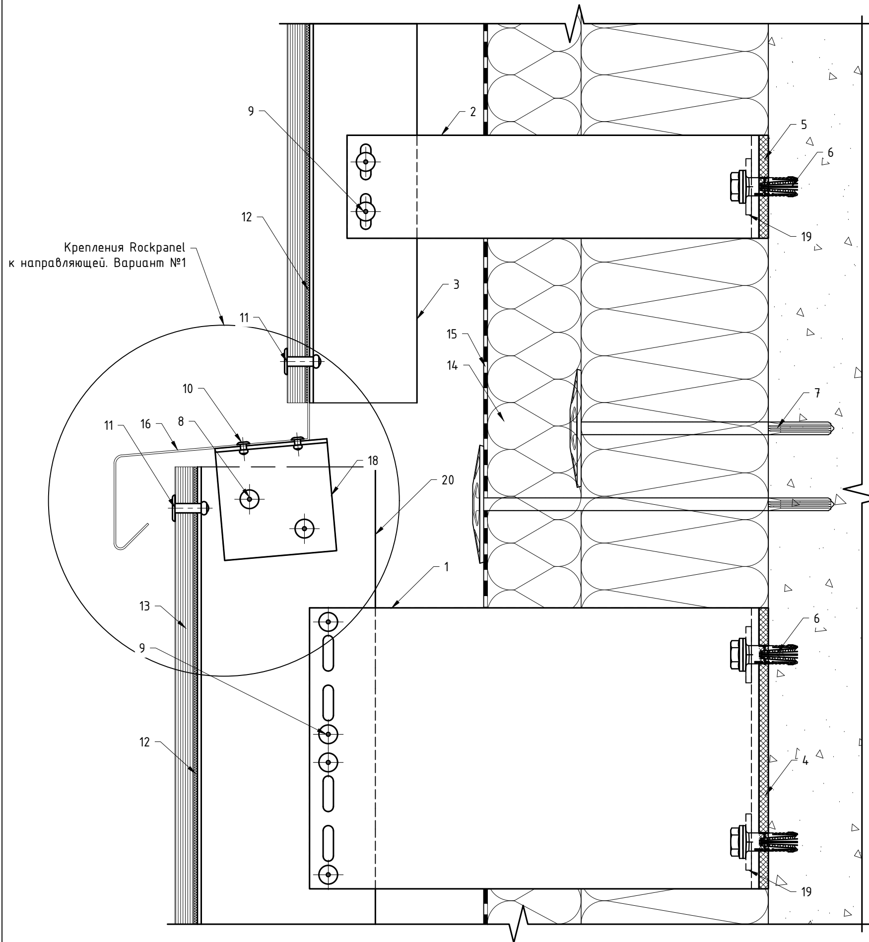
Организация перепада плоскостей облицовки: вариант №1.
