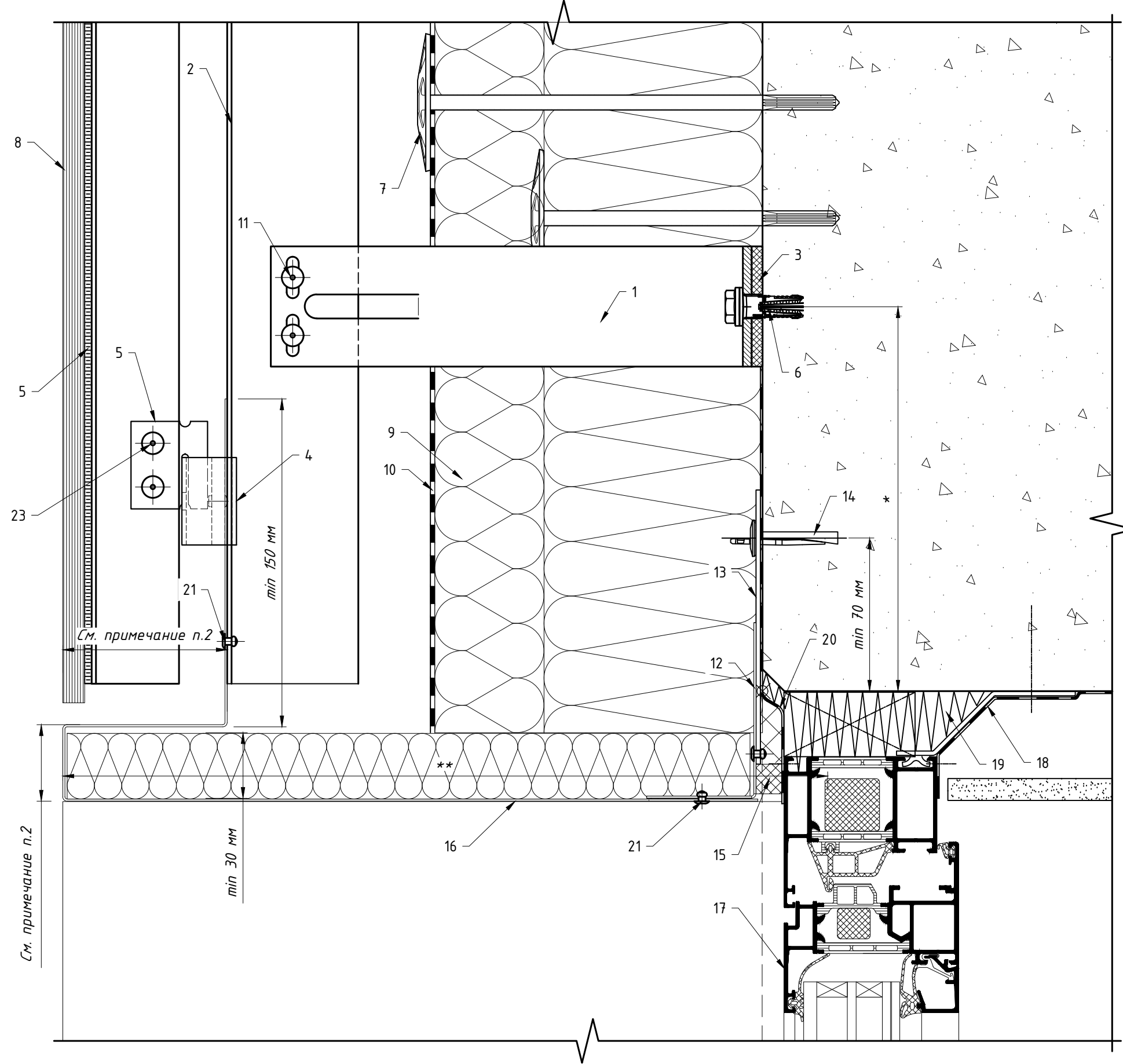
7.4 Примыкание к верхнему откосу: для оконного (дверного) блока установленного в проем, вариант №1. Крепление Rockpanel к направляющей: вариант 3.
