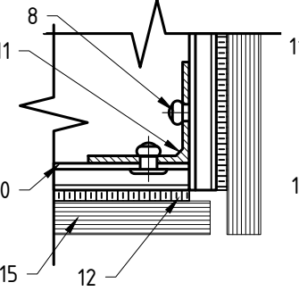
Крепление Rockpanel: вариант №3*** (скрытое крепление, клей и клеящая лента)
