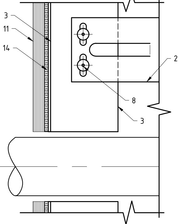
Крепление Rockpanel: вариант №3 (скрытое крепление, клей и клеящая лента)
