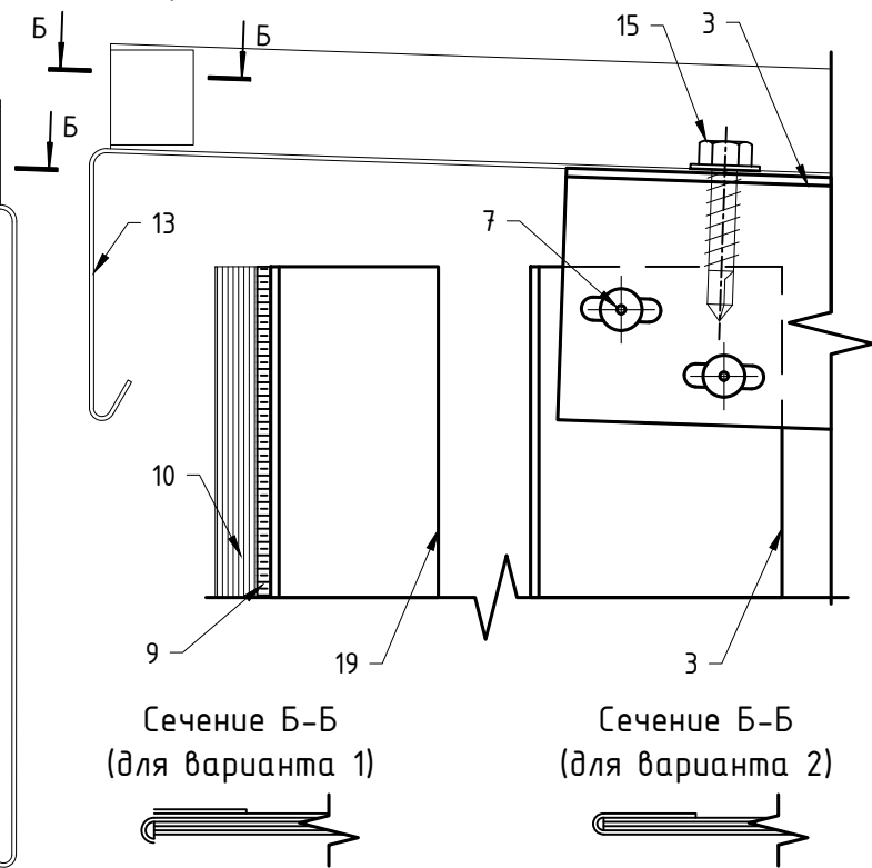
Вариант крепления парапетной крышки №2
