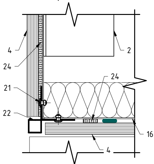
Вариант крепления Rockpanel к направляющей №2
