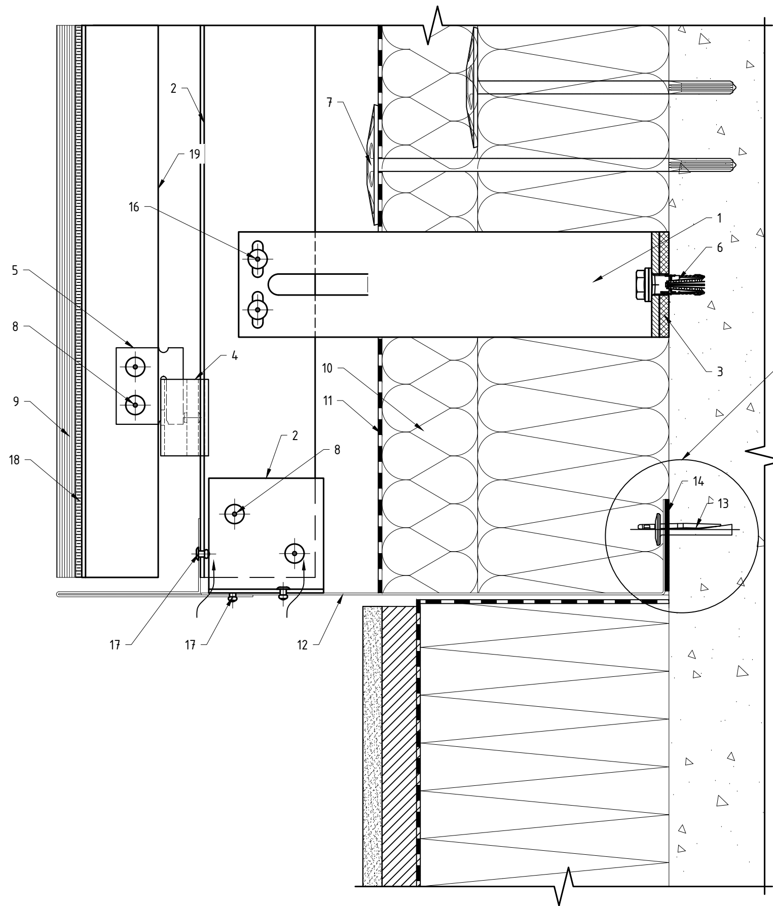
Вариант крепления отлива №1
