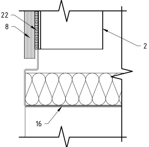
Вариант крепления Rockpanel к направляющей №2
