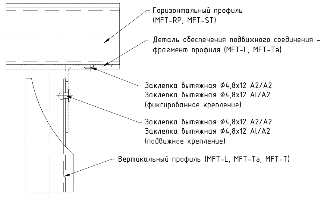
Узел №2 (увеличено)
