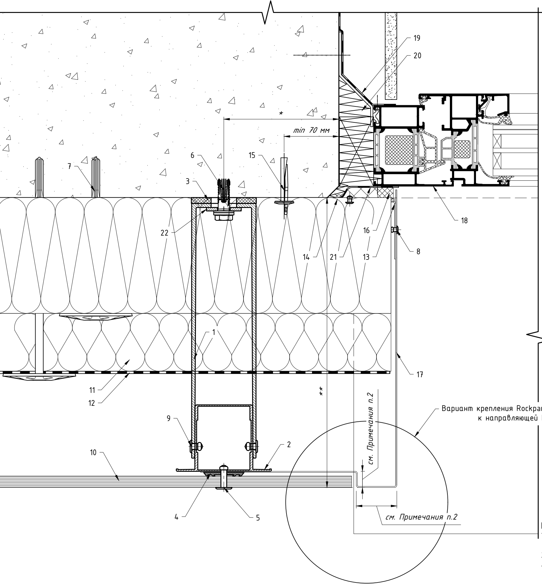
Примыкание к доковому откосу: для оконного (дверного) блока установленного в проем, вариант №1.
