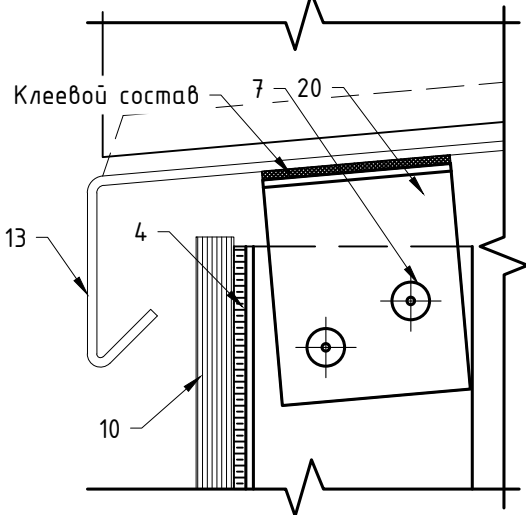
Вариант крепления отлива к направляющей №3
