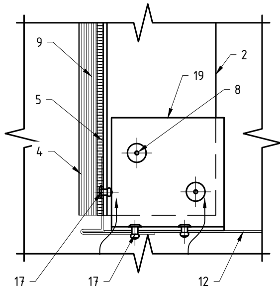
Крепление Roskrapel к направляющей: вариант №2 (скрытое крепление, клей и клеящая лента)
