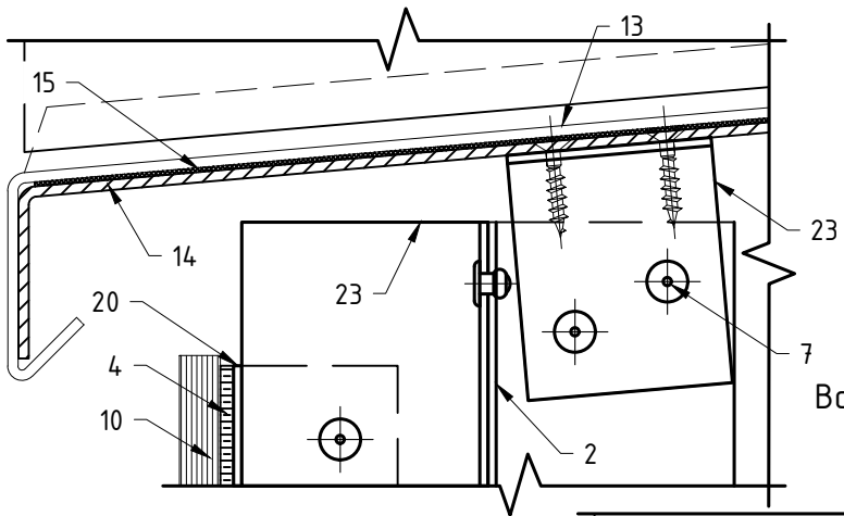
Вариант крепления отлива к направляющей №2
